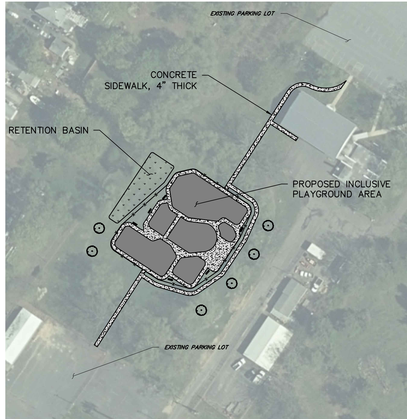
CONCEPT PLAN N.T.S.
