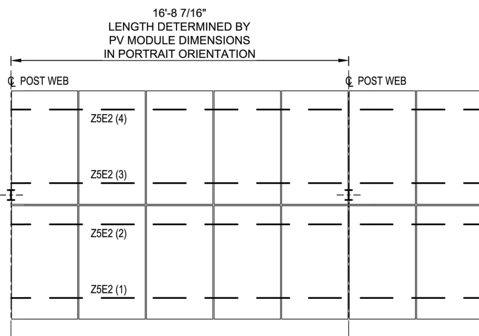
A3 5E2P2 SCALE: 1/4" = 1'-0" BAY PLAN VIEW
